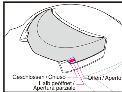
Oberer Lufteinlass / Presa d'aria superiore
